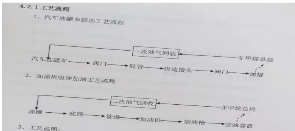
图 4-3 加油站工艺流程图
