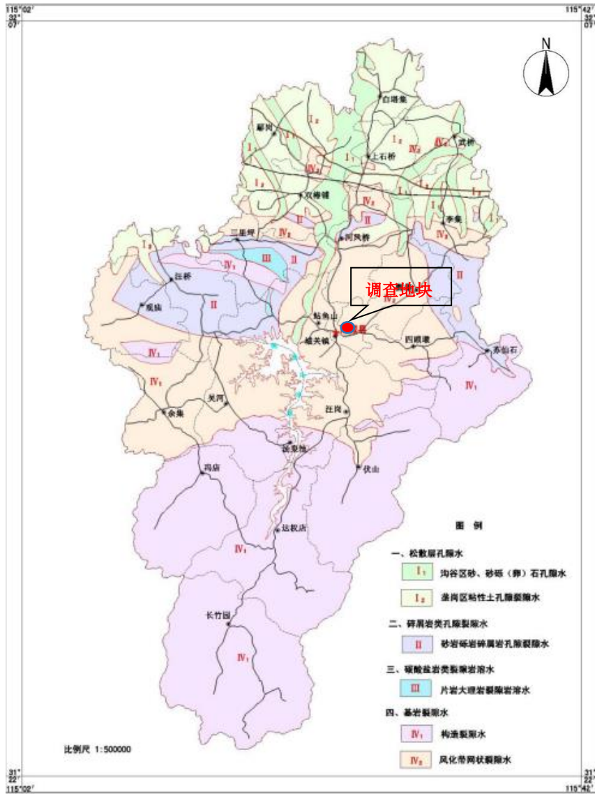
图 3-6 商城县水文地质略图
