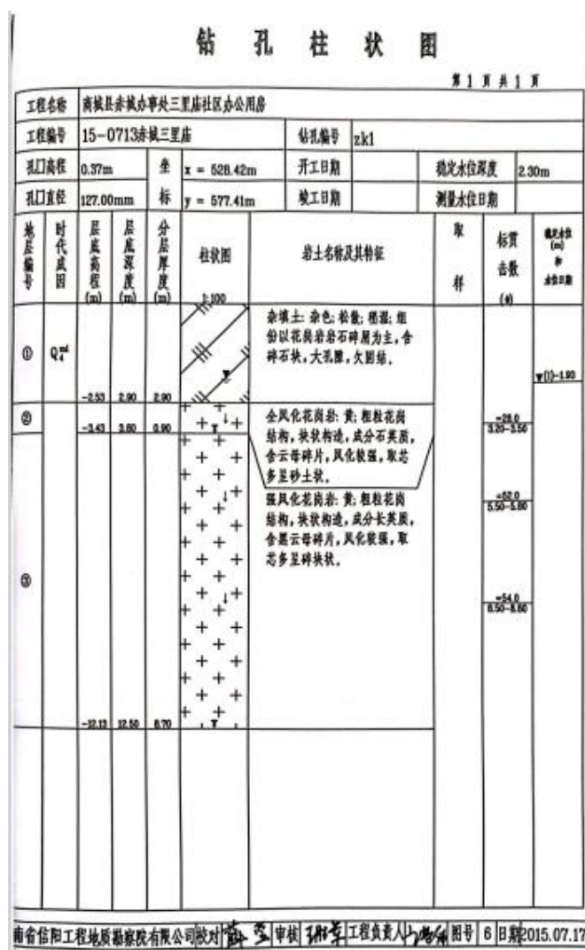
图 3-9 调查地块钻孔柱状图
